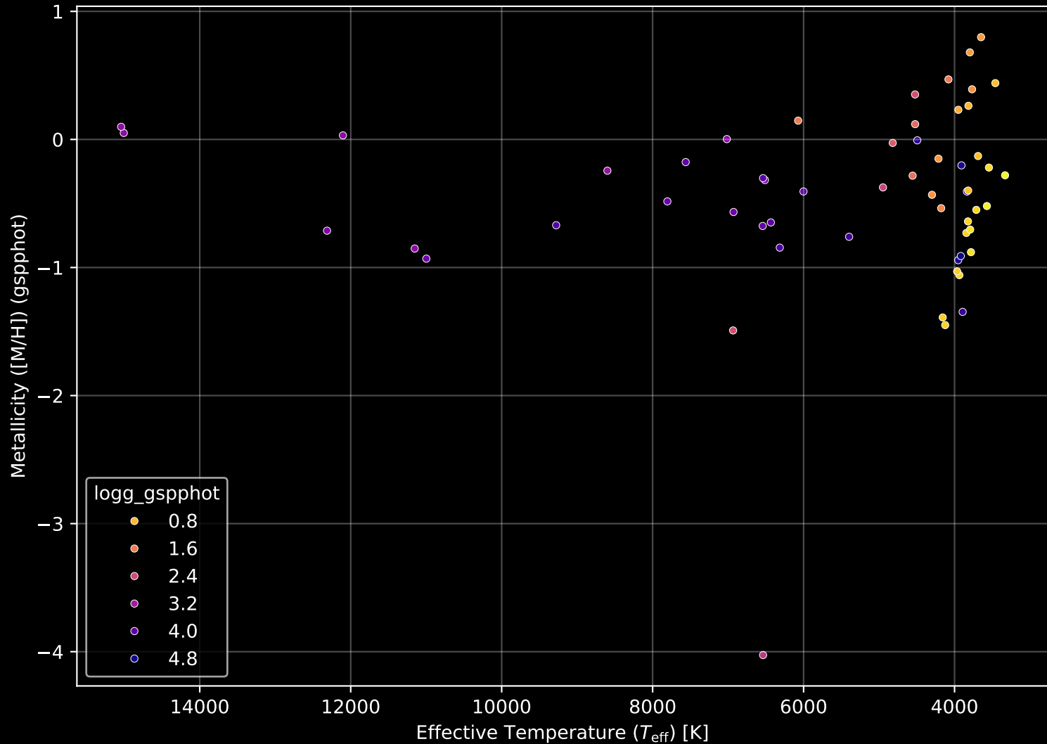
APOGEE DR17 Field: [006+00] Stellar Population Parameters (n= 57)
